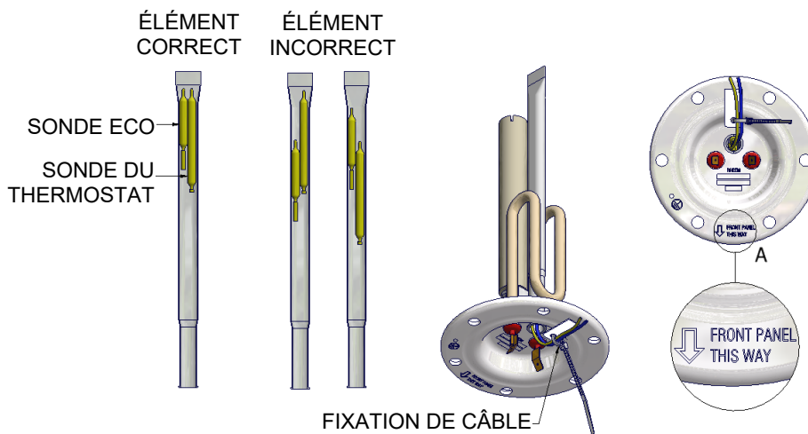
Diagramme. POSITION ADÉQUATE DES SONDES DE TEMPÉRATURE DANS LE PUIT DE L'ÉLÉMENT
