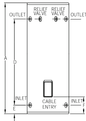
RHEEM 25L-125L
