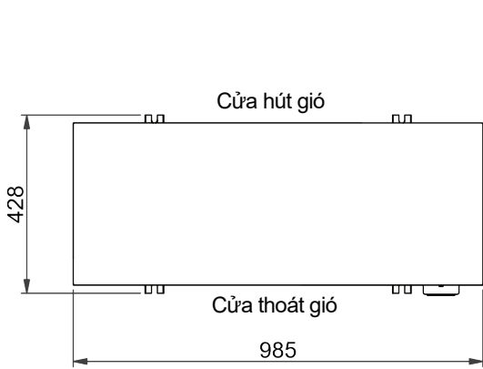
Hình chiếu bằng
